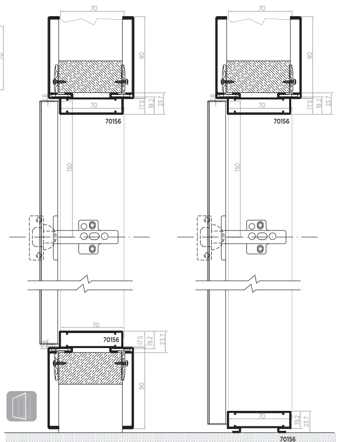
SECCIÓN TRANSVERSAL CON TAPAJUNTAS INFERIORES SECÇÃO TRANSVERSAL COM TAPA-JUNTAS INFERIORES
