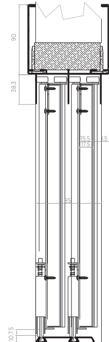
SECCIÓN TRANSVERSAL SIN TAPAJUNTAS INFERIORES SECÇÃO TRANSVERSAL SEM TAPA-JUNTAS INFERIORES
