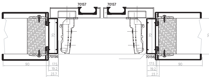
SECCIÓN LONGITUDINAL 2 HOJAS SECÇÃO LONGITUDINAL 2 FOLHAS
