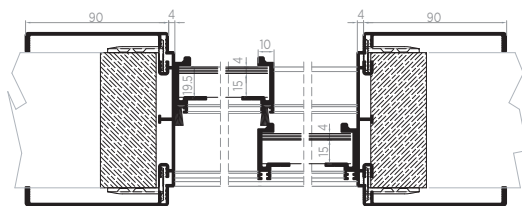
SECCIÓN LONGITUDINAL ESPEJO SECÇÃO LONGITUDINAL EPELHO
