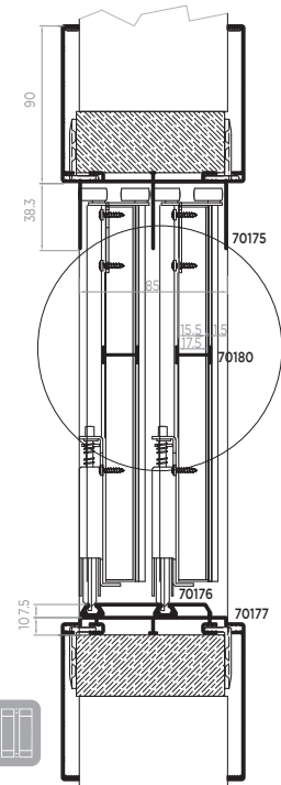
SECCIÓN TRANSVERSAL PANEL JAPONÉS SECÇÃO TRANSVERSAL PAINEL JAPONÉS
