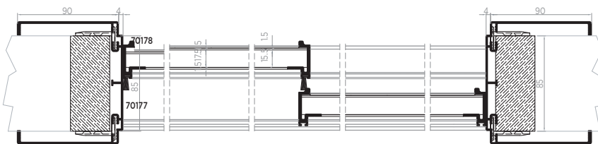
SECCIÓN LONGITUDINAL PANEL JAPONÉS SECÇÃO LONGITUDINAL PAINEL JAPONÉS
